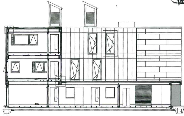
Longitudinal section
